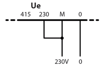
ПОДКЛЮЧЕНИЕ -230V
